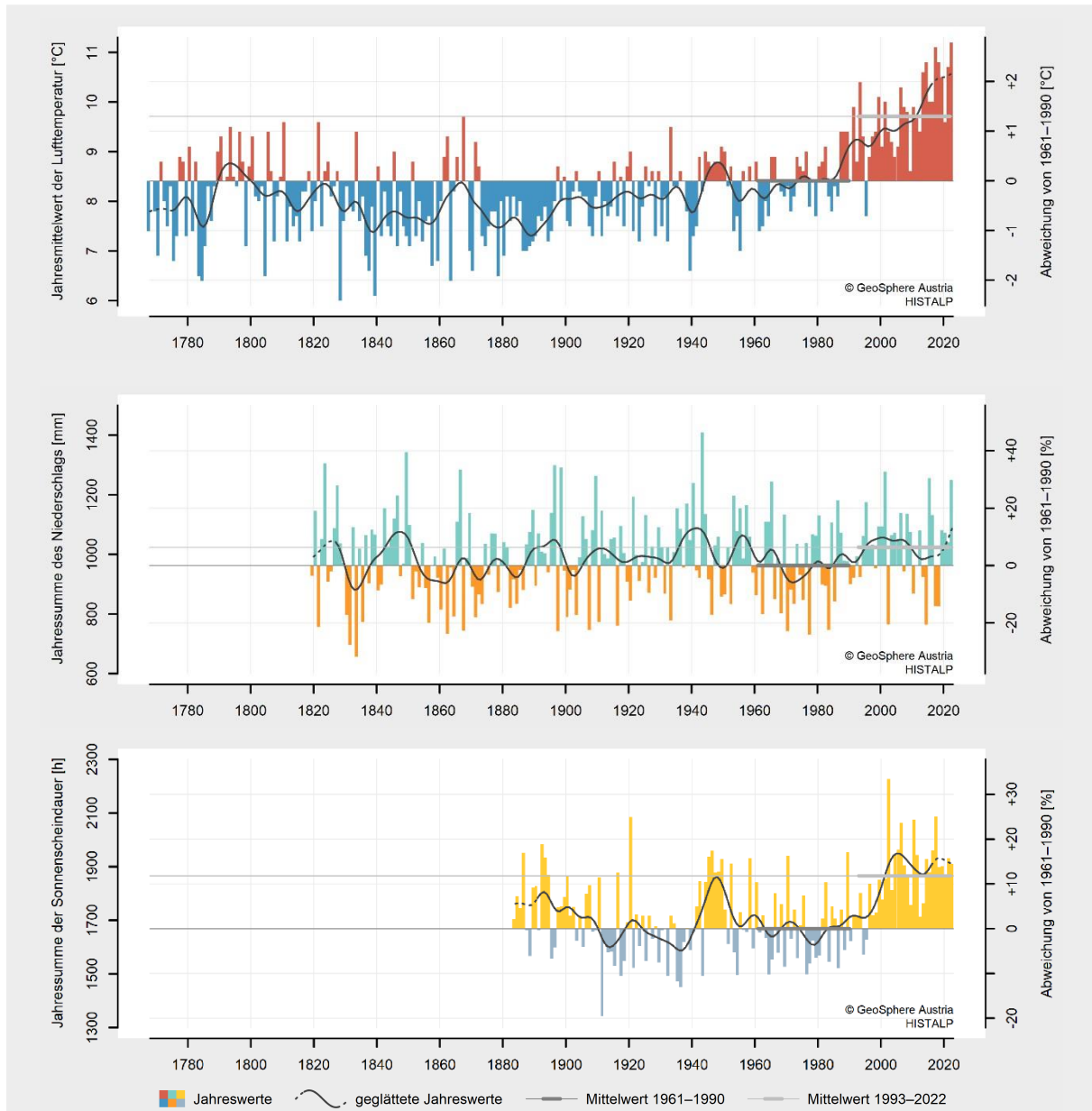
Abbildung 8: Langfristige Entwicklung der Jahreswerte von Lufttemperatur (oben), Niederschlags-summe (Mitte) und Sonnenscheindauer (unten) in Kremsmünster vom Beginn instrumenteller Messungen bis 2023. Die Niveaus der Mittelwerte des Bezugszeitraumes 1961–1990 bzw. der letzten 30 Jahre 1993–2022 sind als dunkelgraue bzw. hellgraue Linien eingetragen.
