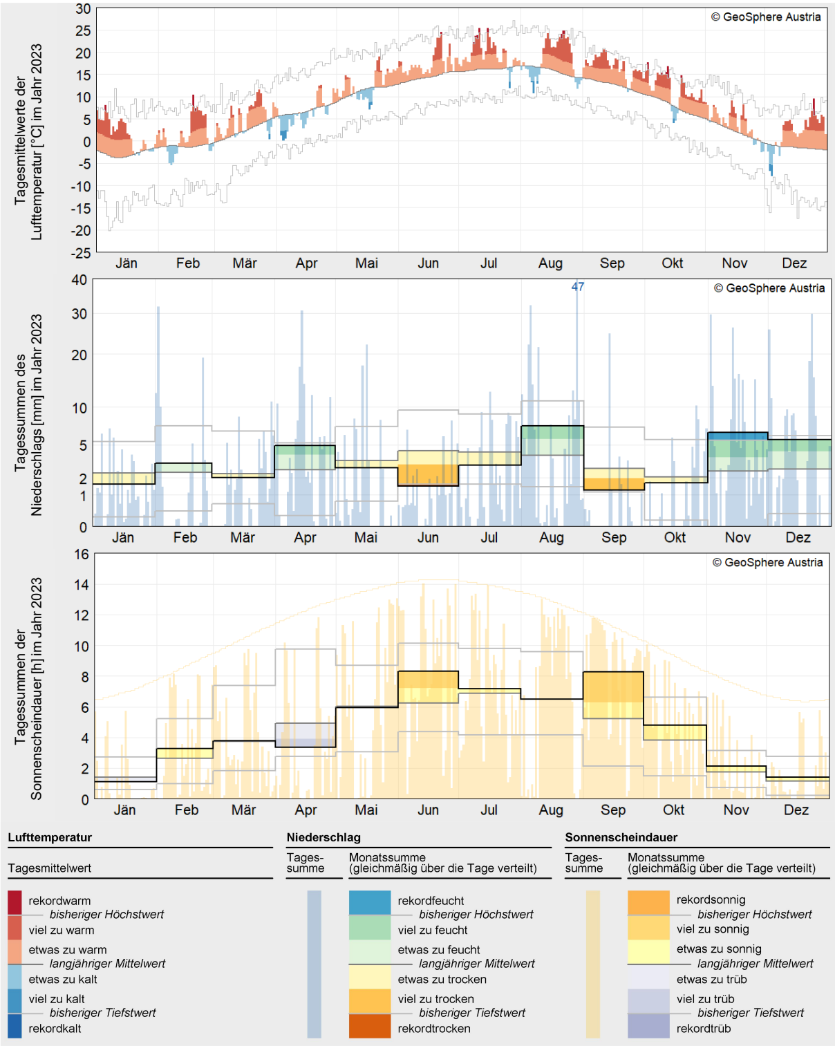
Abbildung 3: Verläufe von täglicher Lufttemperatur, Niederschlagssumme und Sonnenscheindauer im Jahr 2023 in Bezug auf die Mittelwerte des Zeitraumes 1961–1990. Angegeben sind Flächenmittelwerte über Oberösterreich.
